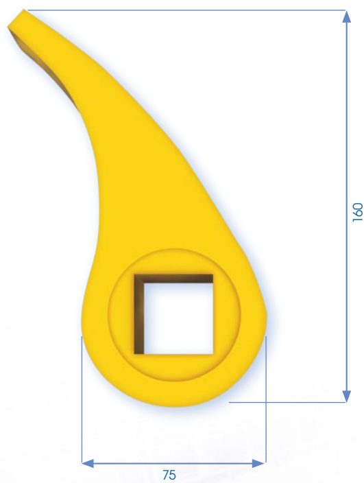
skrobak 8 szerokość modułu: 110 mm
