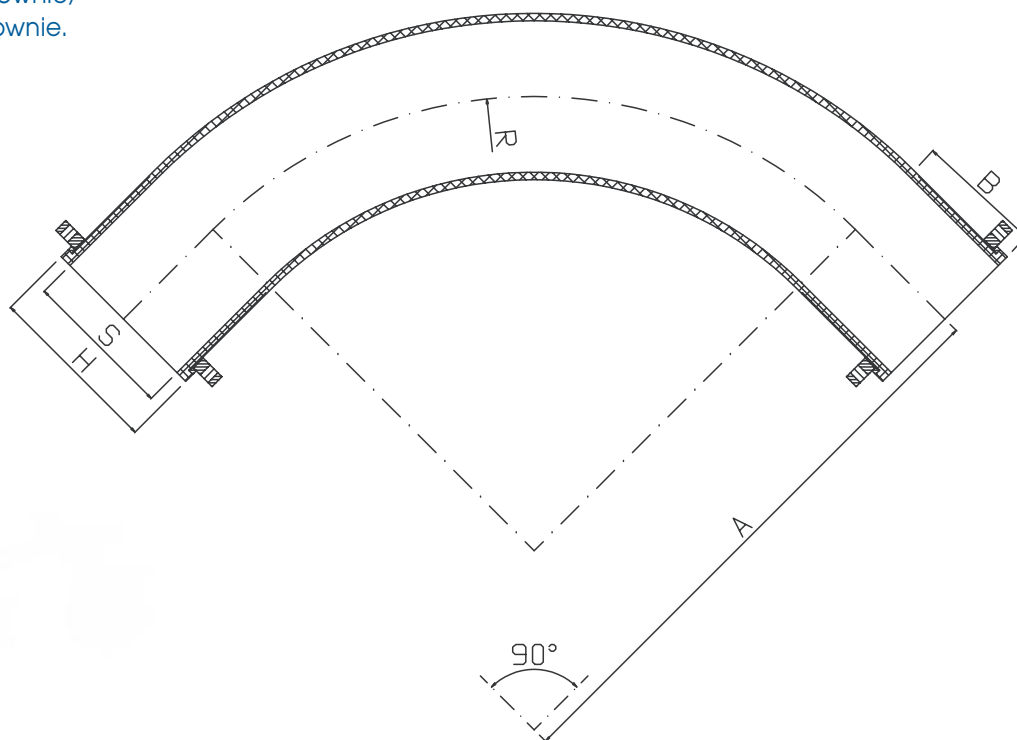
KOLANA L-PUR POLIUTERANOWE Z KOŁNIERZAMI OBROTOWYMI – WYMIARY
